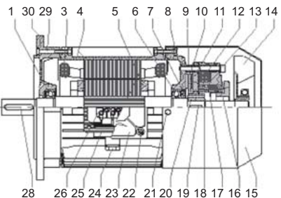
B5 132~160
