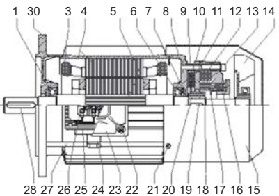
B5 63~112
